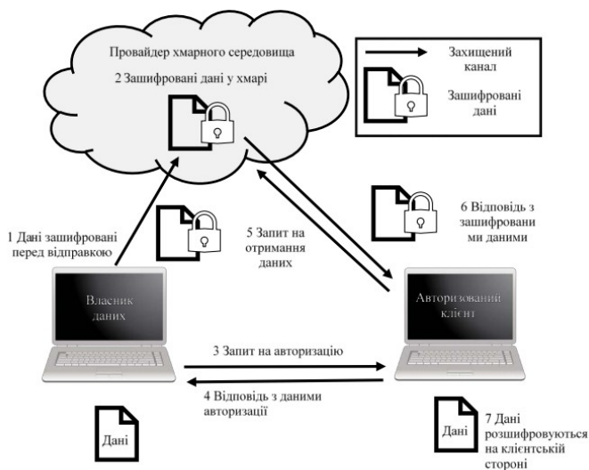
Рис. 1. Варіант механізму шифрування для надійного доступу до персональних даних у хмарі
